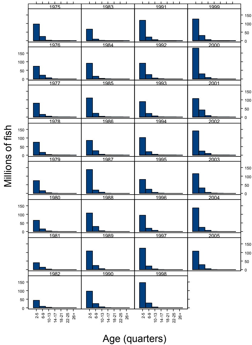
FIGURE B.1. Estimated numbers of yellowfin tuna present in the EPO on 1 January of each year. FIGURA B.1. Número estimado de atunes aleta amarilla presentes en el OPO el 1 de enero de cada año.
