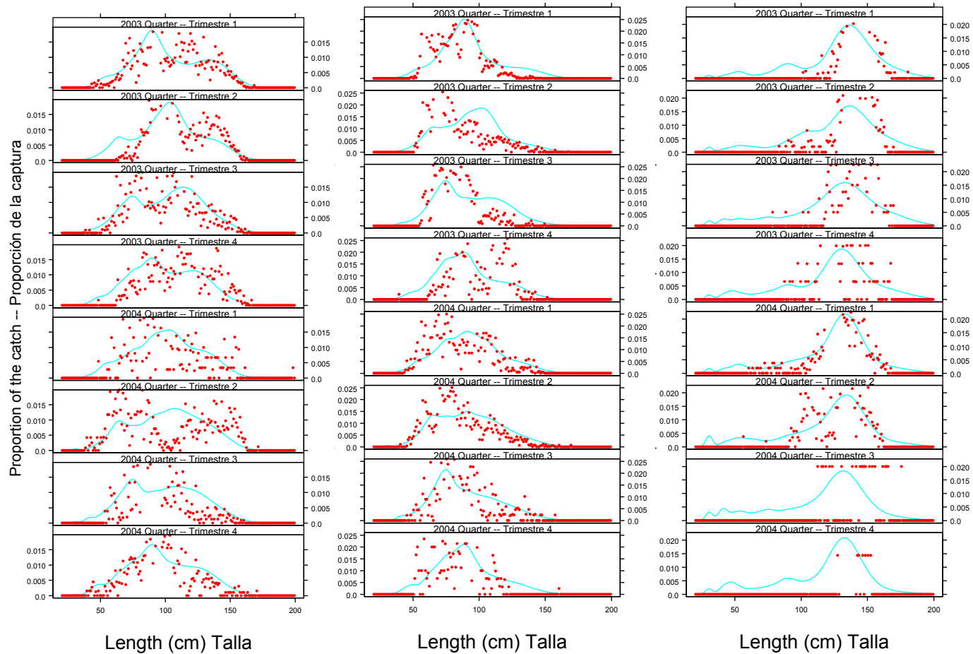
FIGURE 4.8c. Observed (dots) and predicted (curves) size compositions of the recent catches of yellowfin tuna by the fisheries that take tunas in association with dolphins (Fisheries 7-9). FIGURA 4.8c. Composiciones por tamaño observadas (puntos) y predichas (curvas) de las capturas recientes de atún aleta amarilla por las pesquerías que capturan atún en asociación con delfines (Pesquerías 7-9).
