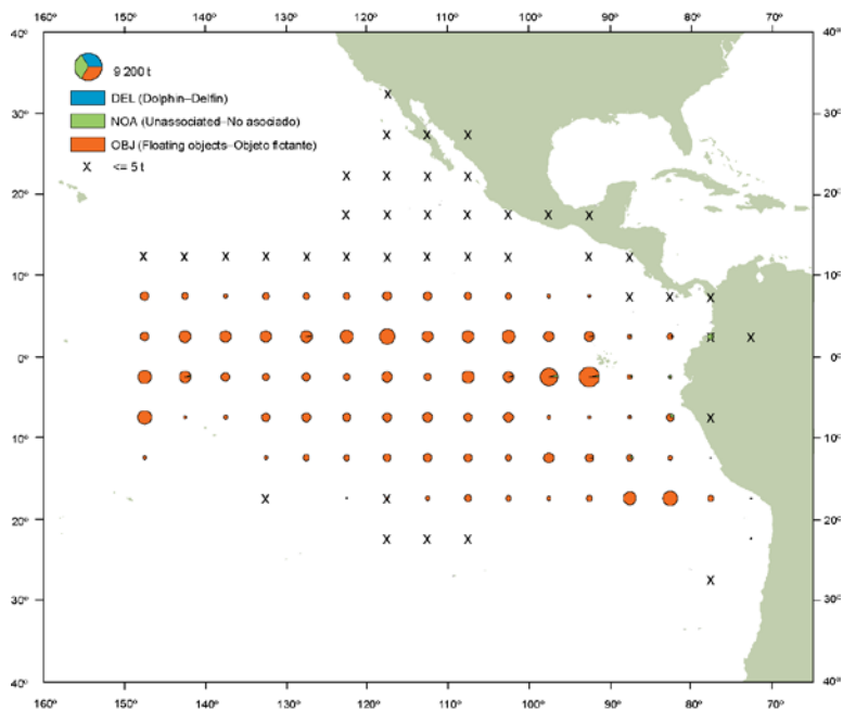
FIGURE A-3b. Annual distributions of the purse-seine catches of bigeye, by set type, 2011. The sizes of the circles are proportional to the amounts of bigeye caught in those 5° by 5° areas. FIGURA A-3b. Distribución anual de las capturas cerqueras de patudo, por tipo de lance, 2011. El tamaño de cada círculo es proporcional a la cantidad de patudo capturado en la cuadrícula de 5° x 5° correspondiente.
