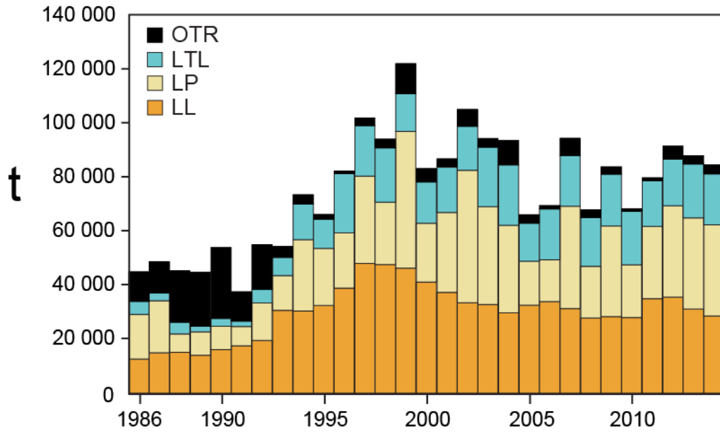
FIGURE F-1a. Retained catches of North Pacific albacore. FIGURA F-1a. Capturas retenidas de albacora del Pacífico norte.
