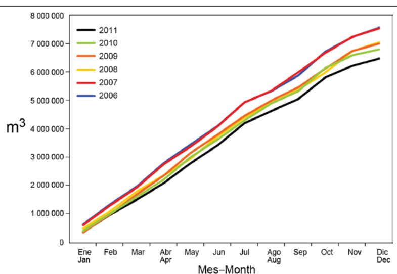
Figura 3. Capacidad acumulativa de la flota cerquera y cañera en el mar, por mes, 2006-2011
