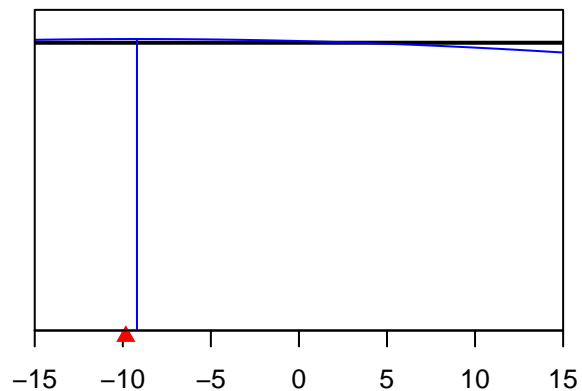
Size_DbIN_top_logit_A5-LL-n(5)
