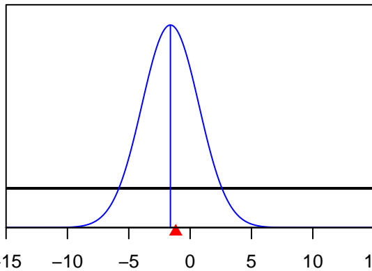
Size_DbIN_top_logit_A3-LL-n(3)
