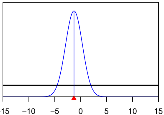
Size_DbIN_top_logit_A4-LL-n(4)
