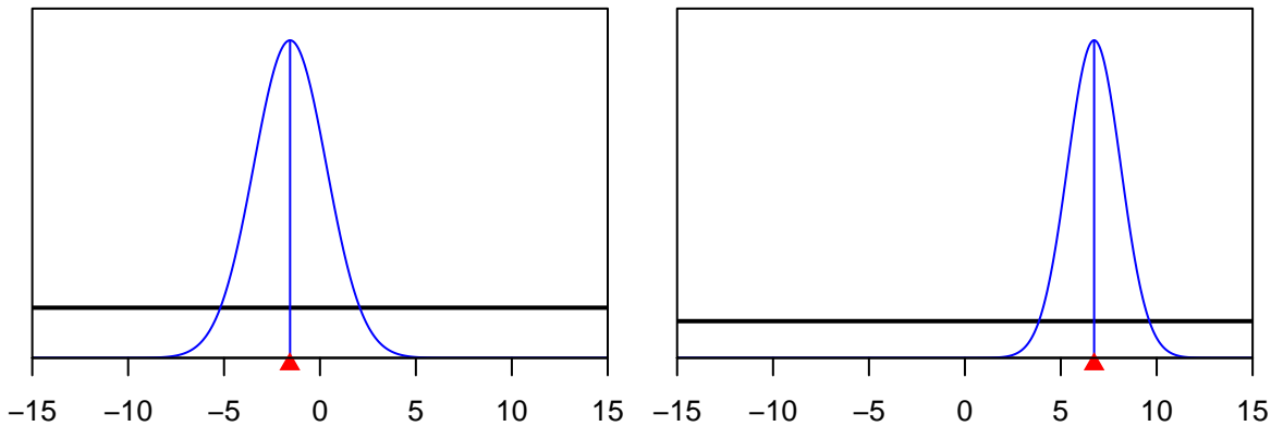
Size_DbIN_top_logit_A6-OBJ(17)
