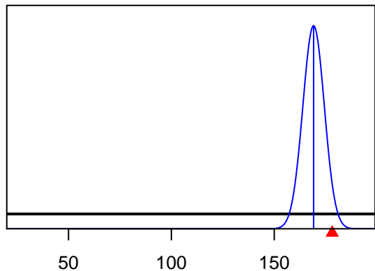
Size_DbIN_top_logit_A2-LL-n(2)_BLK2repl_17
