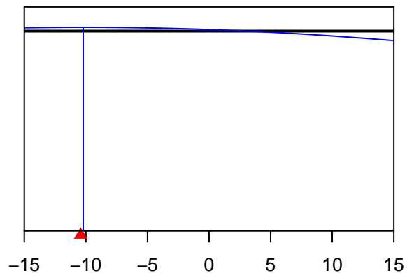
Size_DbIN_top_logit_A2-LL-n(2)_BLK2repl_17
