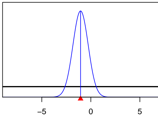
SizeSpline_Val_8_F4-Obj_Cc_Q14(4)
