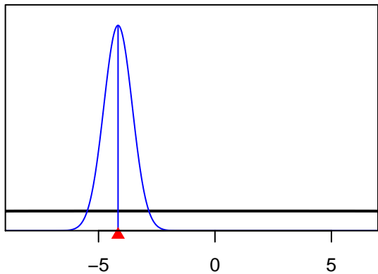
SizeSpline_Val_2_F22-BB(22)
