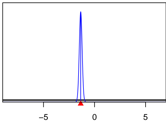
SizeSpline_Val_3_F11-NOA_N(11)
