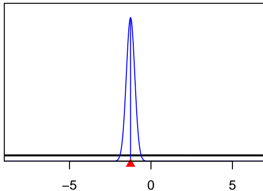
SizeSpline_GradLo_F7-Obj_Nc_Q23(7)
