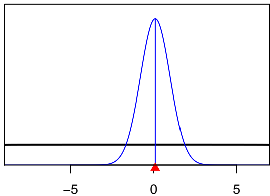
SizeSpline_Val_9_F10-Obj_S_Q23(10)
