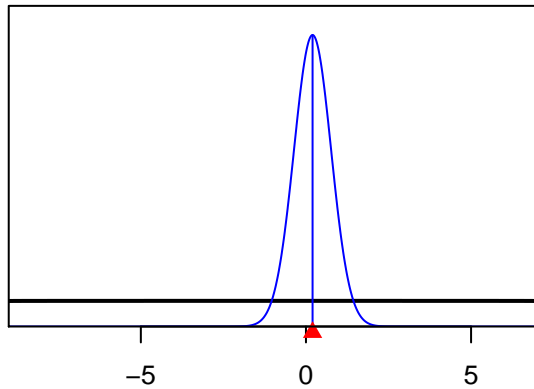
SizeSpline_Val_5_F5-Obj_S_Q14(5)
