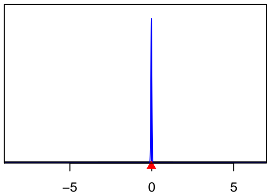
SizeSpline_Val_6_F11-NOA_N(11)
