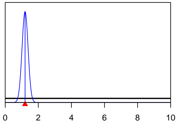
SizeSpline_GradLo_F12-NOA_C(12)
