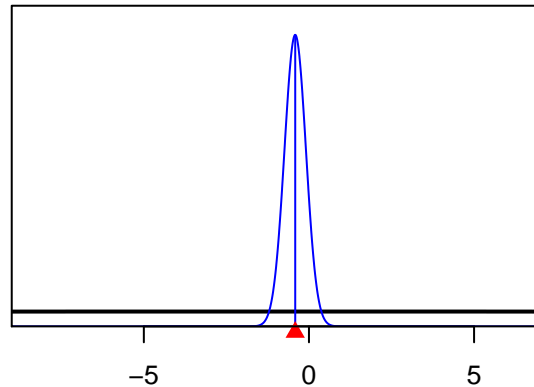
SizeSpline_Val_6_F8-Obj_C_Q23(8)
