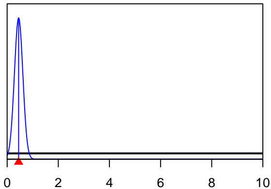
SizeSpline_GradLo_F17-DEL_M(17)
