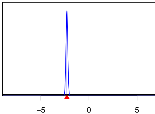
SizeSpline_Val_2_S1-PS_DEL_VAST(41)
