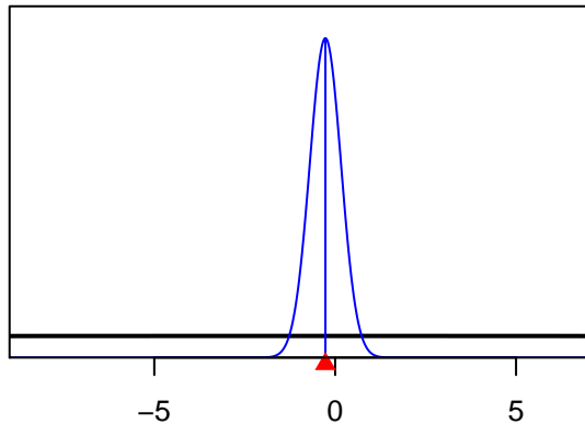
SizeSpline_Val_10_F8-Obj_C_Q23(8)
