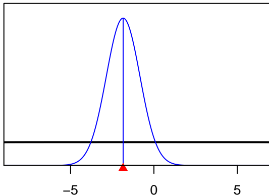
SizeSpline_GradLo_F2-Obj_Nc_Q14(2)
