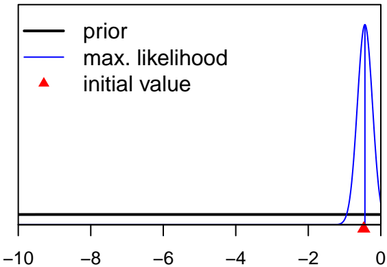
SizeSpline_Val_2_F7-OBJ_Nc_Q23(7)
