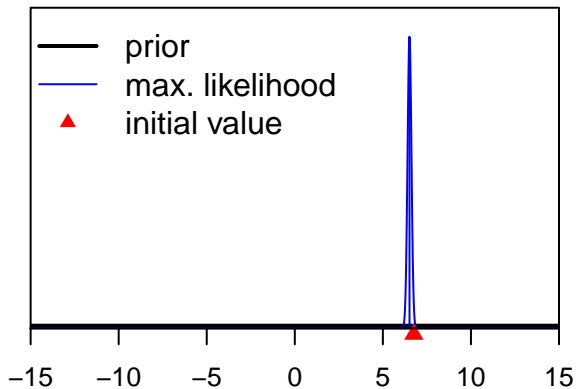
SizeSpline_GradLo_F22-BB(22)
