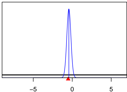
SizeSpline_Val_5_F16-DEL_NE(16)
