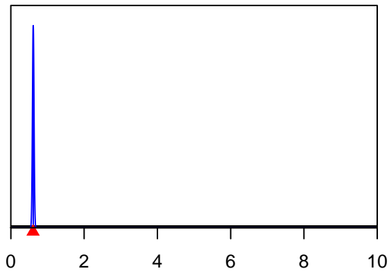
SizeSpline_GradLo_S1-PS_DEL_VAST(41)
