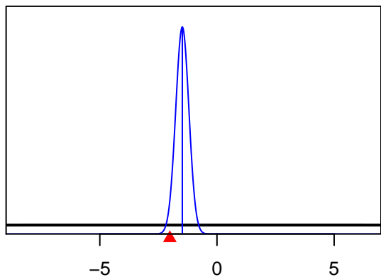
SizeSpline_Val_3_F16-DEL_NE(16)
