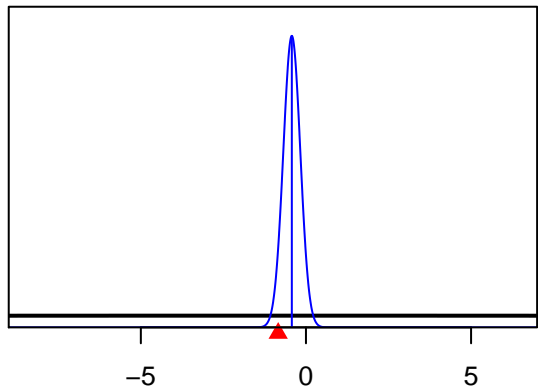
SizeSpline_Val_5_F16-DEL_NE(16)
