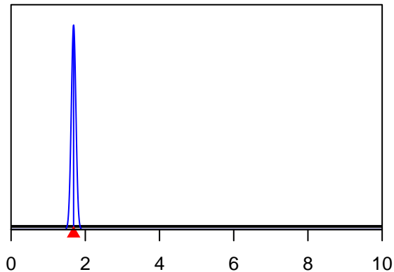
SizeSpline_GradHi_F6-Obj_N_Q23(6)
