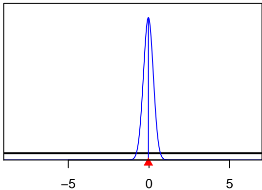
SizeSpline_Val_3_F8-Obj_C_Q23(8)
