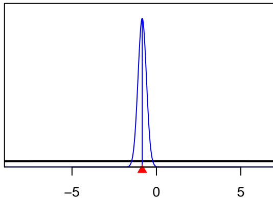
SizeSpline_Val_5_F16-DEL_NE(16)
