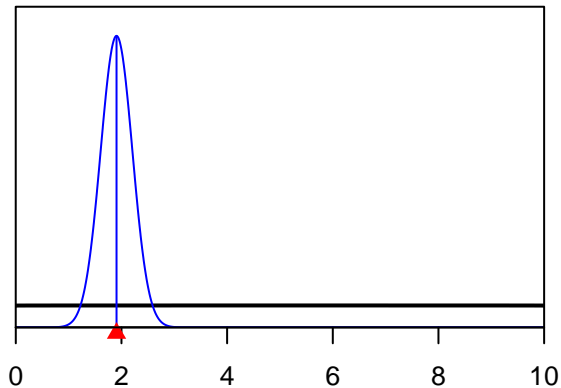
SizeSpline_GradHi_F4-Obj_Cc_Q14(4)
