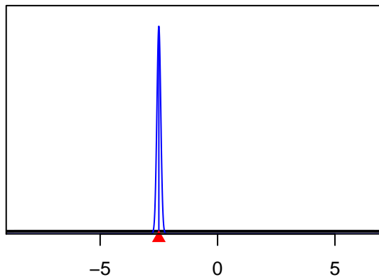
SizeSpline_Val_2_S1-PS_DEL_VAST(41)
