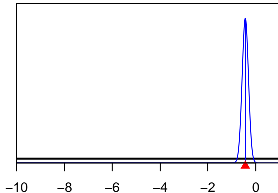
SizeSpline_Val_2_F22-BB(22)
