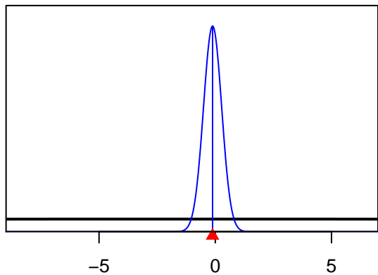
SizeSpline_Val_3_F9-Obj_Cc_Q23(9)
