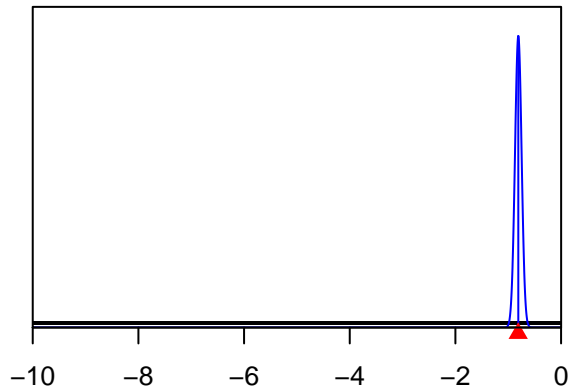
SizeSpline_GradHi_S1-PS_DEL_VAST(41)
