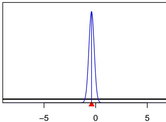
SizeSpline_Val_6_F9-Obj_Cc_Q23(9)
