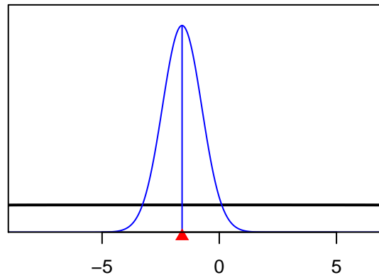
SizeSpline_Val_9_F1-OBJ_N-Q14(1)
