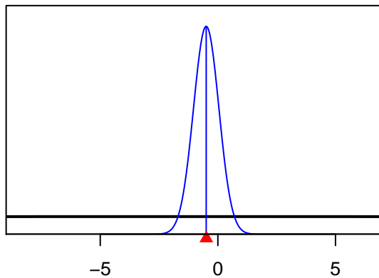
SizeSpline_Val_9_F16-DEL_NE(16)
