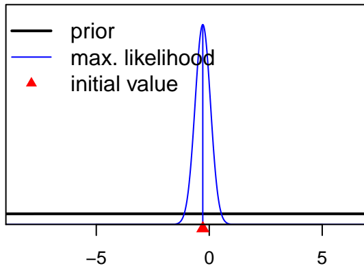
SizeSpline_Val_9_F16-DEL_NE(16)
